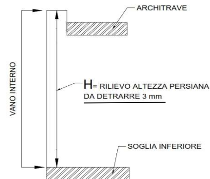
SEZIONE VERTICALE Rilievo altezza
